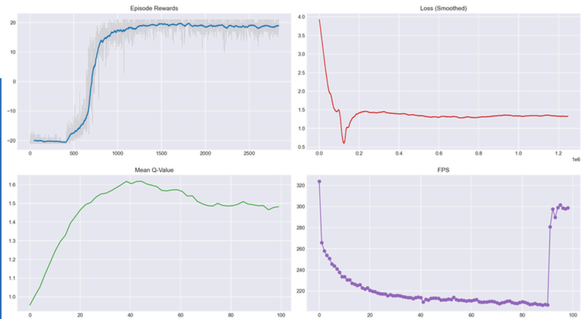
C51 Metrics - 5_LR_1e-4
