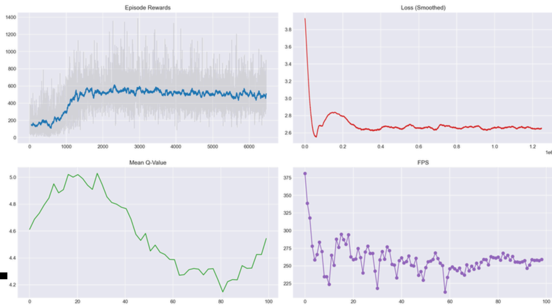
C51 Metrics - 5_LR_1e-4
